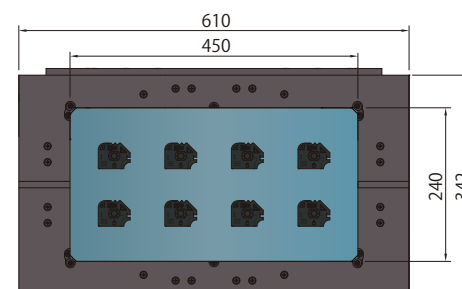
大型ステージを活かした複数個連続測定
