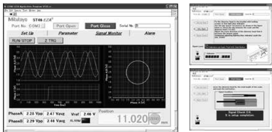
PC画面で信号強度確認・パラメータ設定が可能 (PCは、お客様にてご準備をお願いします)
