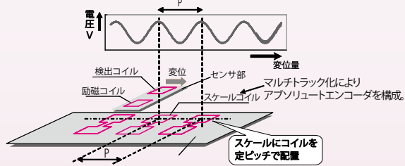
[図2] 電磁誘導式スケールの検出原理
