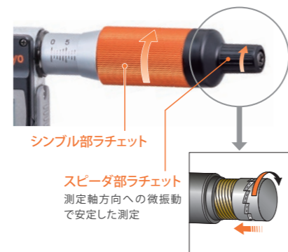
ラチェットシンプル機構
